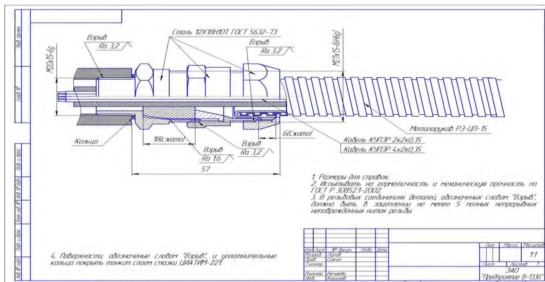
Рис. В3 – Чертеж средств взрывозащиты кабельного ввода
